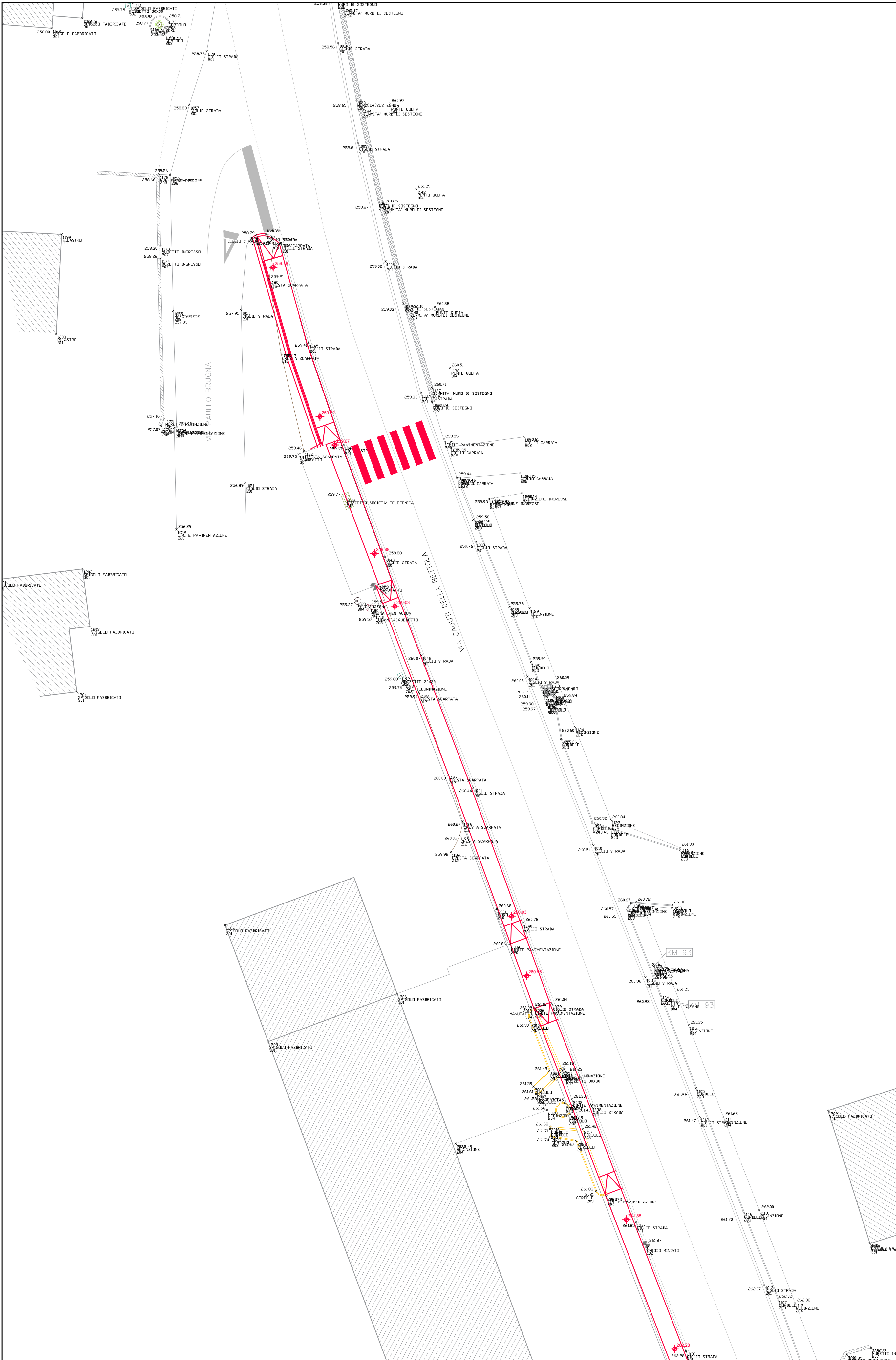
TRATTO D1 - DEMOLIZIONI E COSTRUZIONI - SOLUZIONE 1 - Scala 1:200
