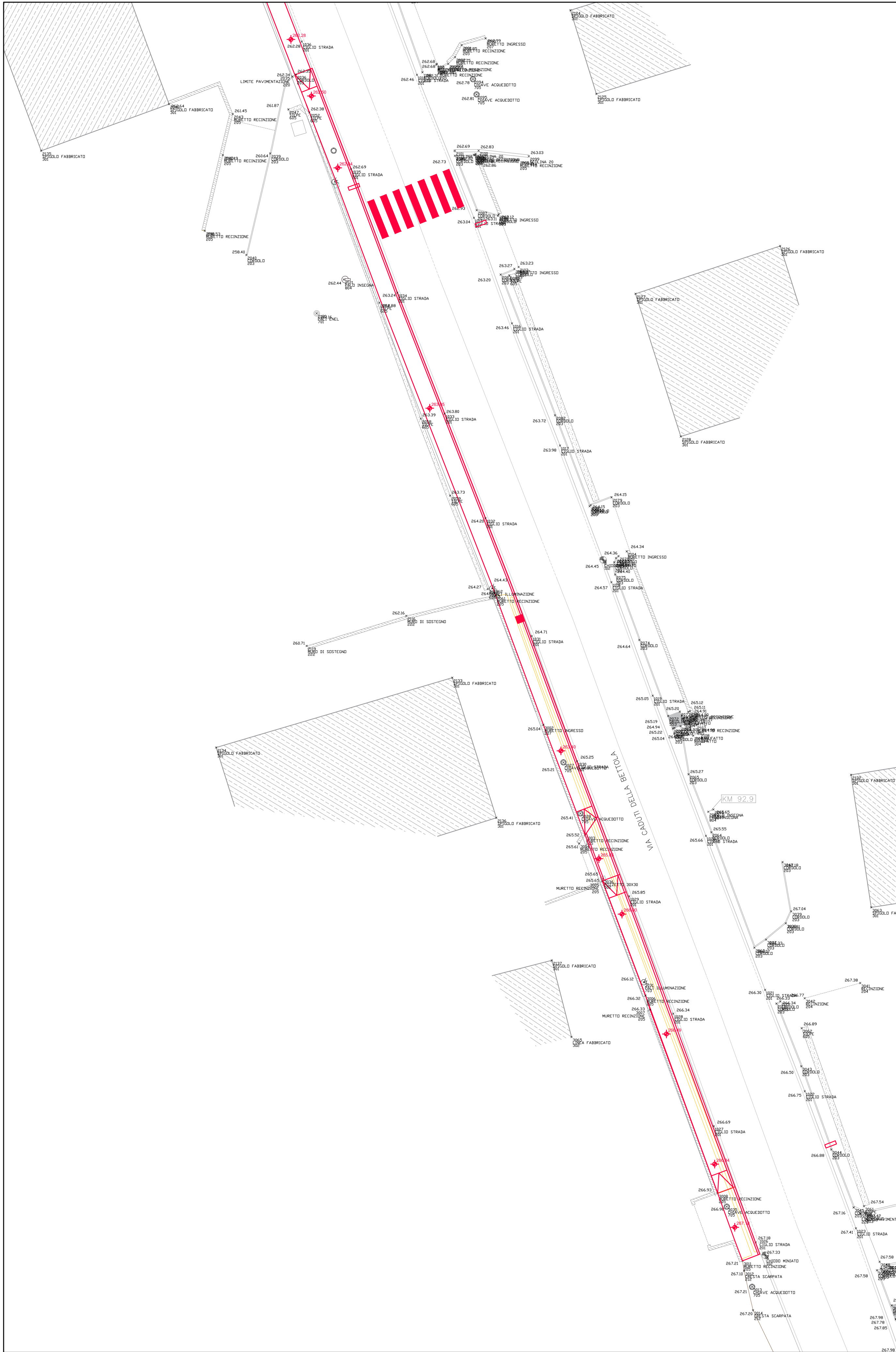
TRATTO D2 - DEMOLIZIONI E COSTRUZIONI - Scala 1:200
