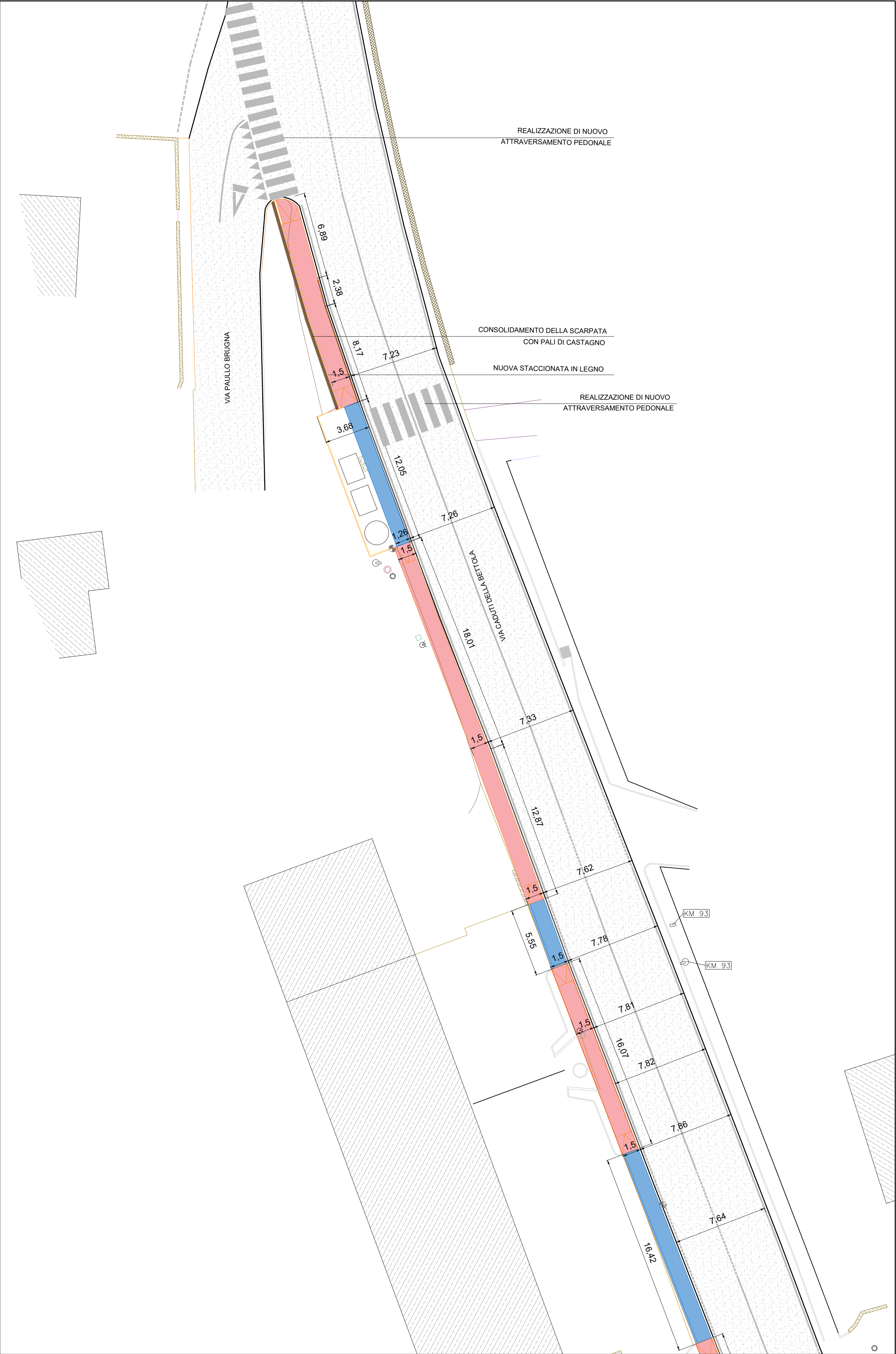
TRATTO D1 - PLANIMETRIA DI PROGETTO - SOLUZIONE 1 - Scala 1:200
